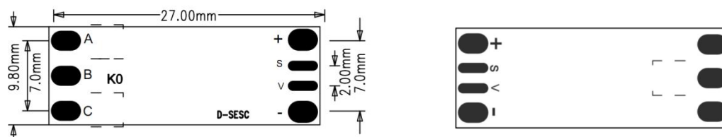
顶层视图
