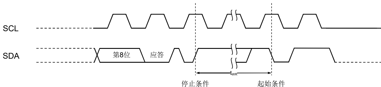
图5 总线时序
