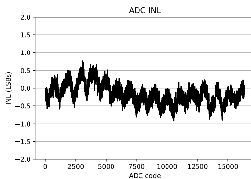
(b) INL
