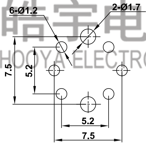
P.C.B LAYOUT
