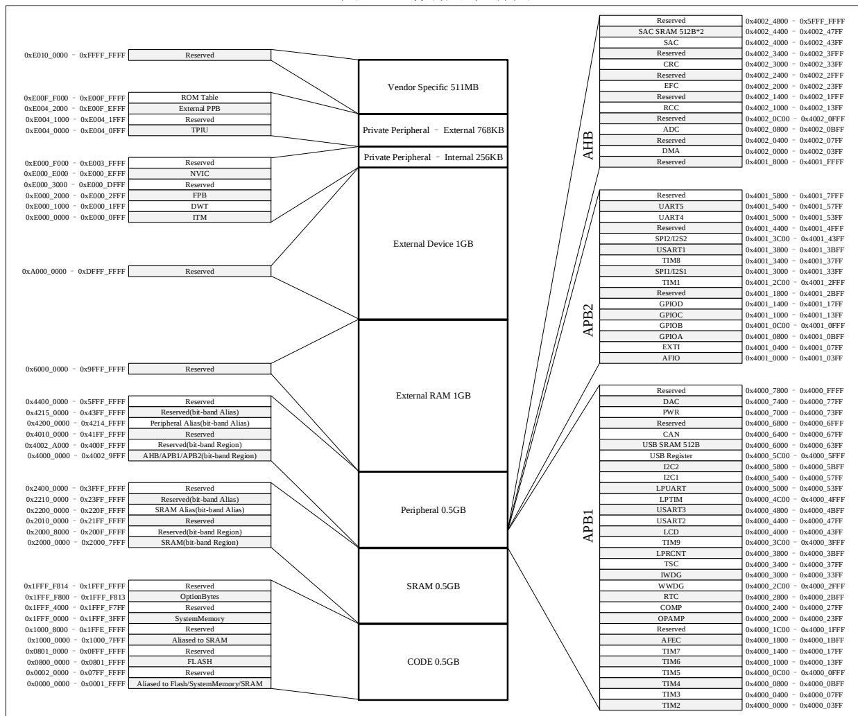
图 2-1 存储器映射图
