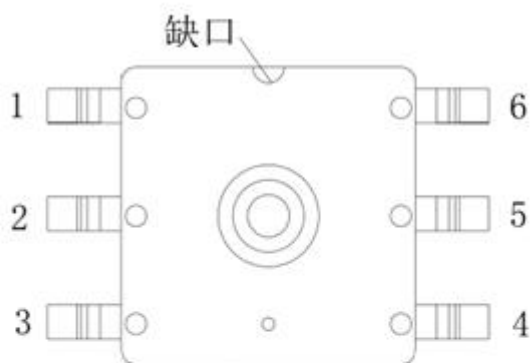
图 3.1 俯视图
